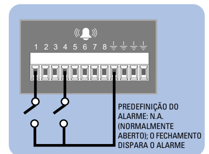
Figura 5. Conexões do alarme
